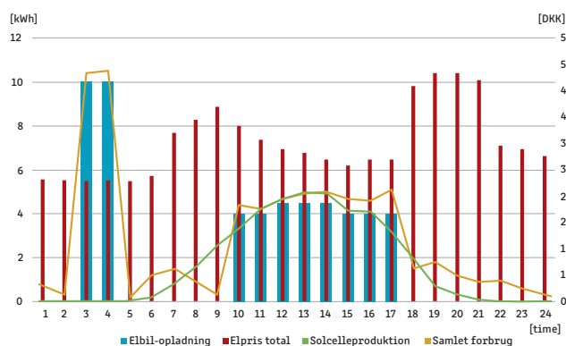
III. 4.2 - Oplad elbilen med strøm enten fra solcellerne om dagen eller køb billig strøm fra elnettet om natten.
