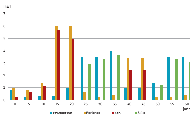
Ill. 5.4 - Viser et eksempel over en time med produktion og forbrug vist med blå og gul. Det som skal købes er vist med rødt og det som skal sælges med grøn.
