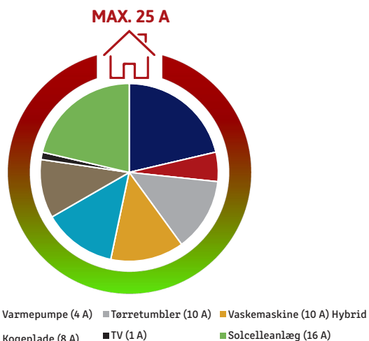
Ill. 6.2 - Belastninger i en almindelig dansk bolig.
